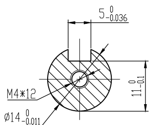
A-A(2:1)
