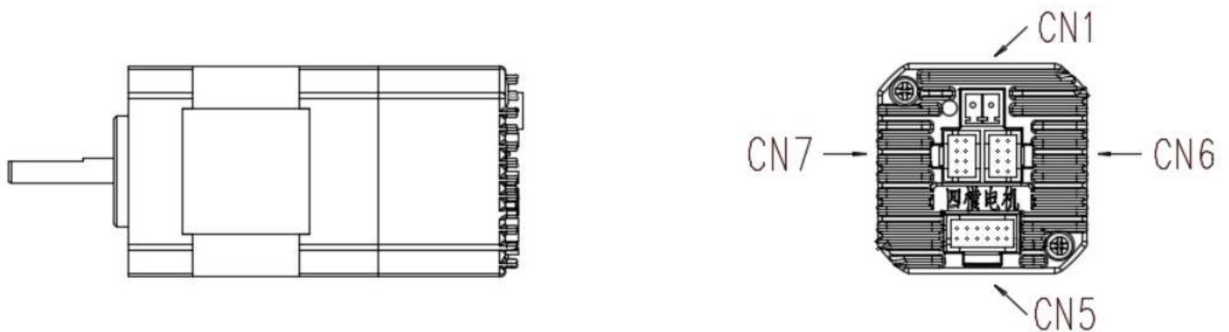
4) 一体式型号: MD42端子接口图
