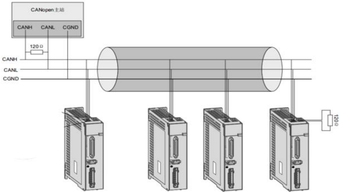
图 2 组网方案 2
