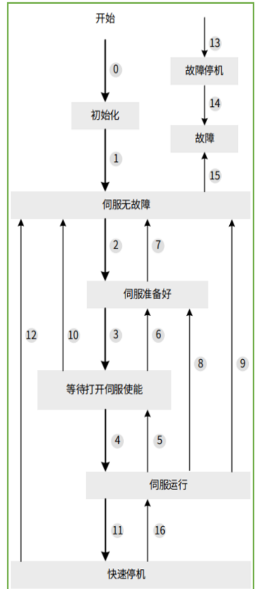
CIA402 状态跃迁图
