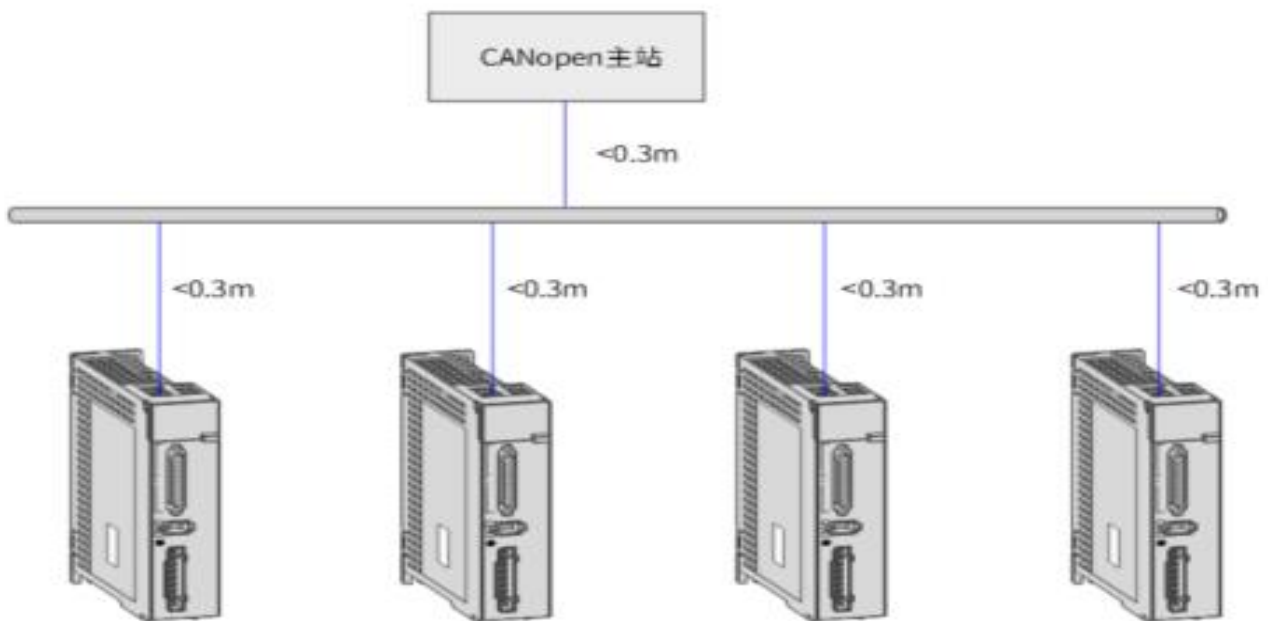
图 1 组网方案 1
