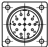
绝对式编码器连接器
