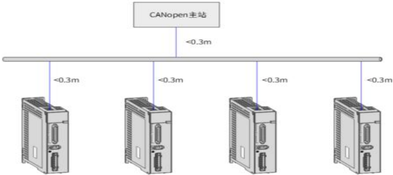
图<组网方案 1>
