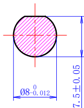
B-B (2:1)
