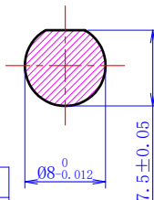
B-B (2:1)
